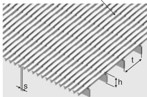
Profil nośny / Supporting profile / Stützdraht / Profil porteur
