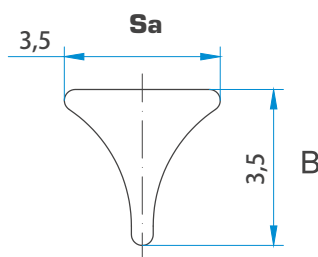
Profil nośny / Supporting profile / Stützdraht / Profil porteur
